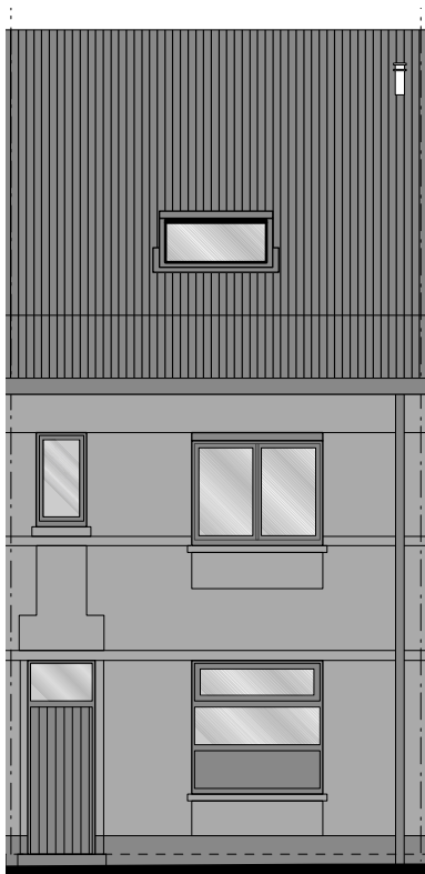
VOORGEVEL
